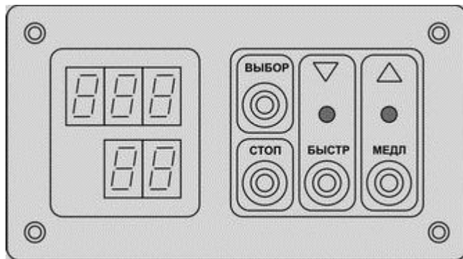
Рисунок 1 Органы индикации и управления БПР08
